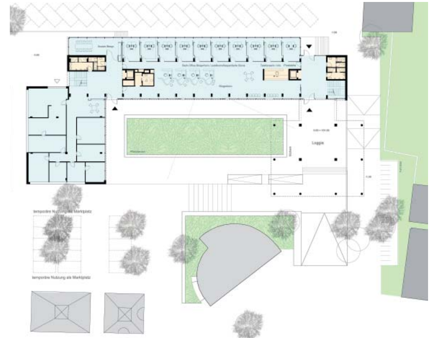
Grundriss Erdgeschoss
